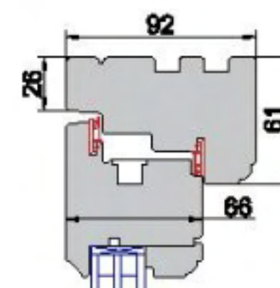
Flush 66/92
