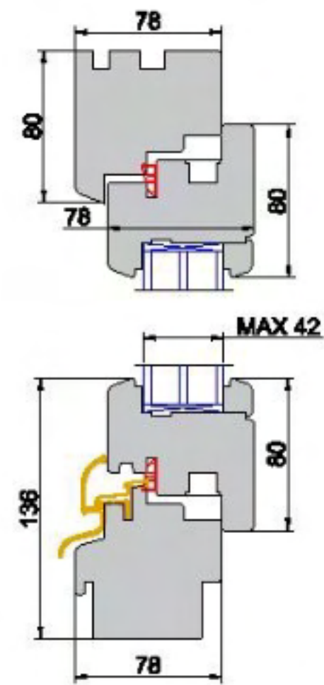
IV 78
