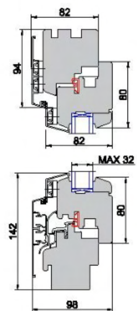
IV 68 Aluclad
