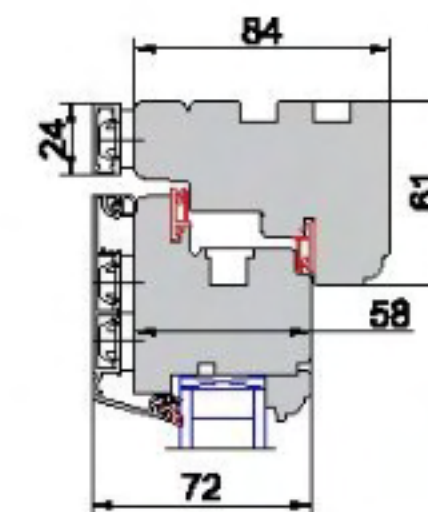
Flush 58/84 Aluclad
