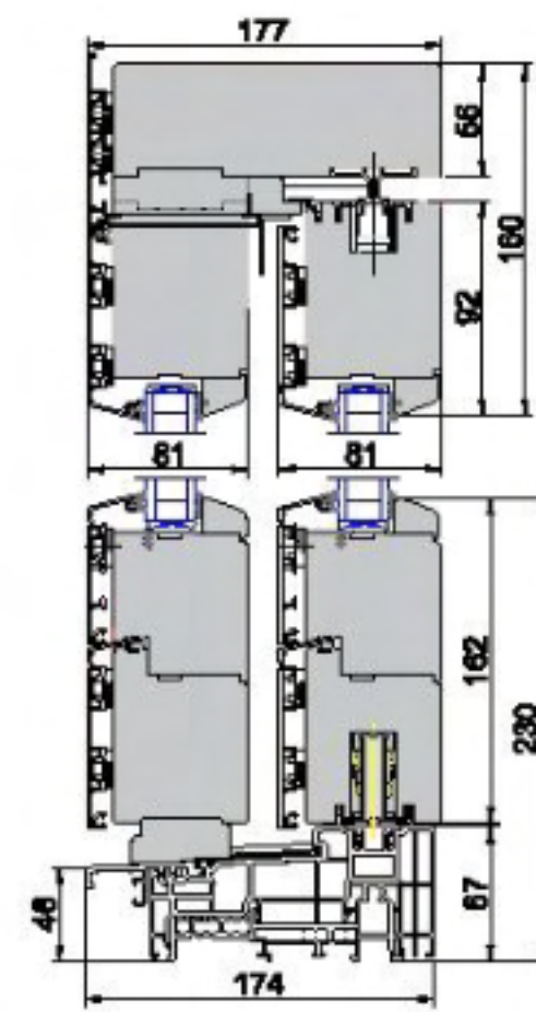
HS 68 Aluclad
